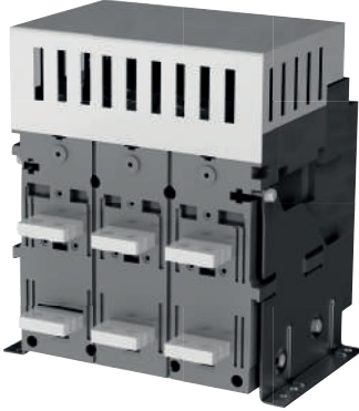
YATAY BAĞLANTI TİPİ
